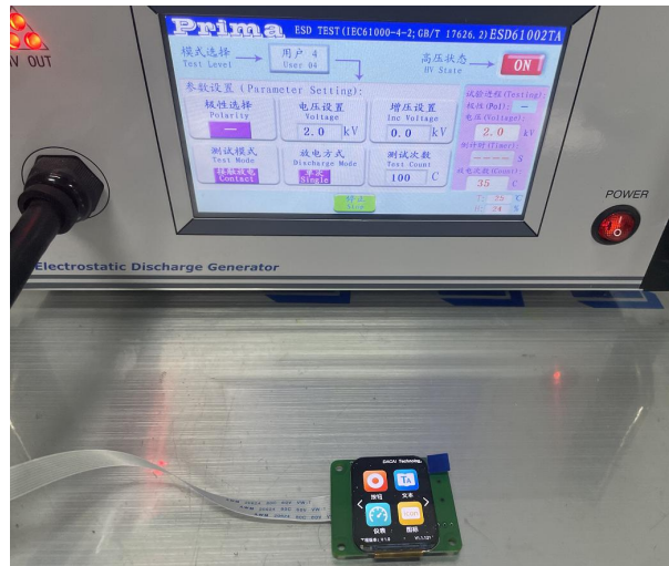
图 4-2 ESD 测试图
