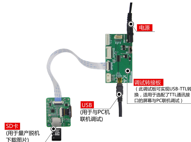
图 1-3 调试工具图
